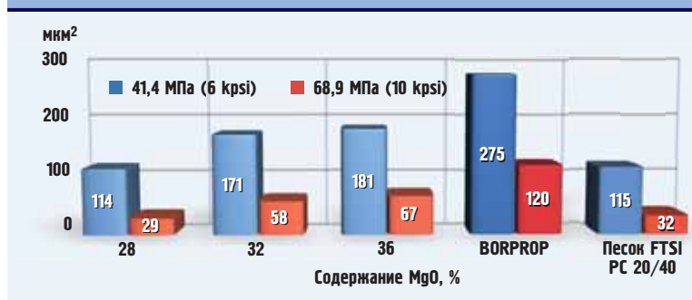
Рис.2 Изменение долговременной проницаемости для магниезно-силикатных и алюмосиликатных пропантов
