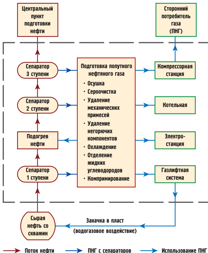
Рис. 1. Рациональное использование попутного газа
